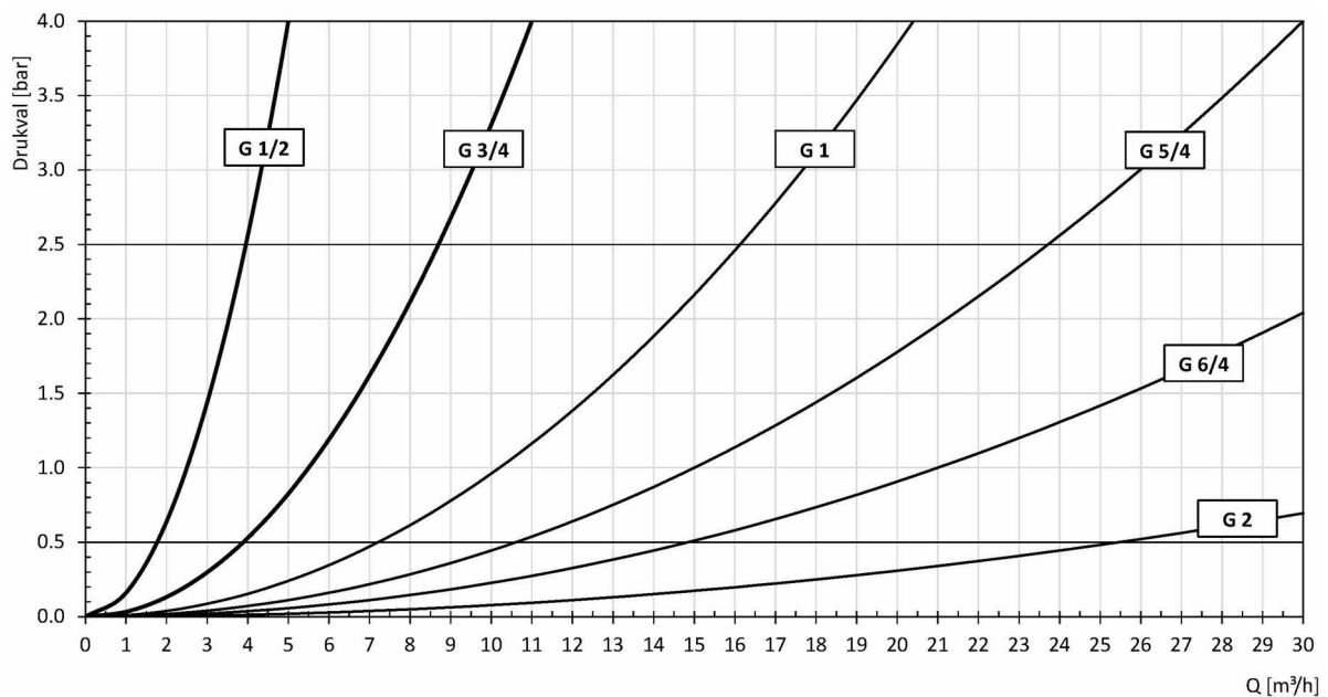
12 Figuur 4: Grafiek doorlaat magneetafsluiters type ACL 107 en ACL 107 BIG
